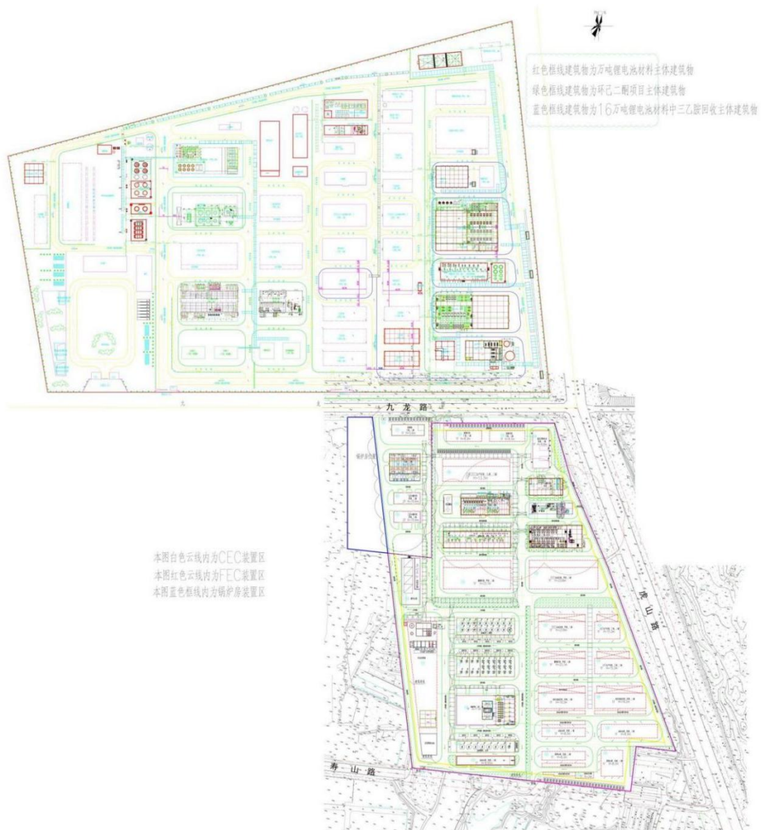
图 4.2 厂区总平面布置图
