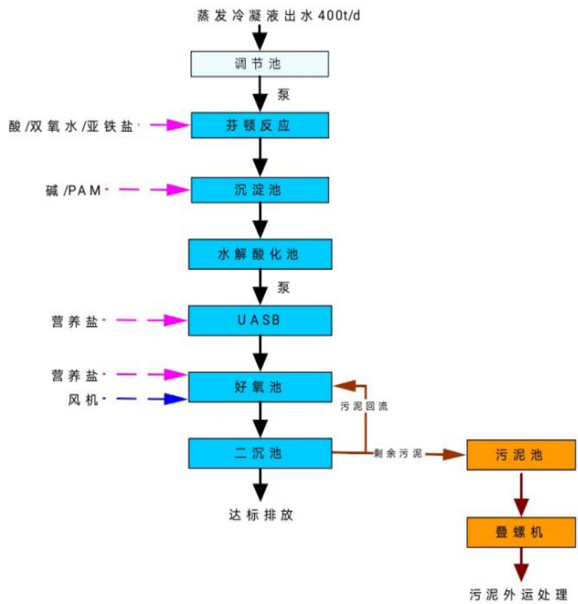
图 4.1-9 污水处理工艺流程图
